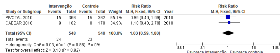
Figura 2 – Metanálise da mortalidade global. EVAR versus acompanhamento clínico, AAA pequenos.
