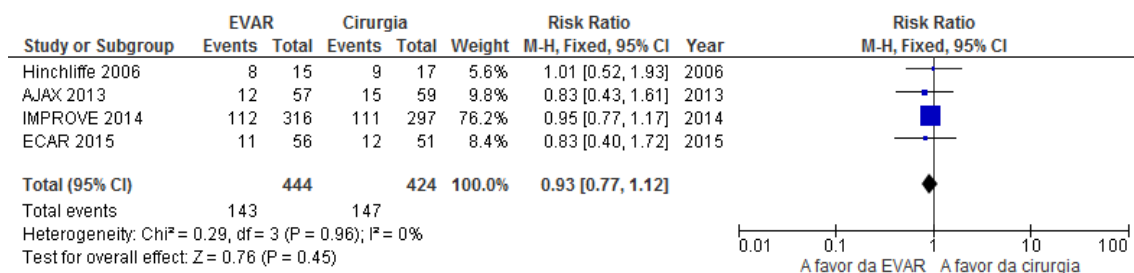
Figura 14 - Metanálise da mortalidade em 30 dias da EVAR versus cirurgia aberta para AAA rotos.
