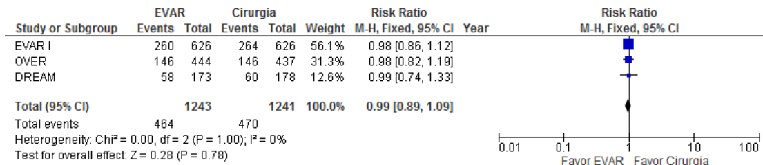
Figura 6 - Mortalidade geral em longo prazo, EVAR versus cirurgia aberta.
